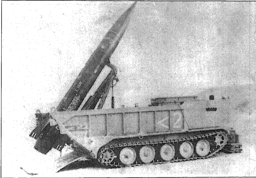
صاروخ أرض أرض مثبت فوق عربة مجنزرة وهو جاهز للانطلاق.
