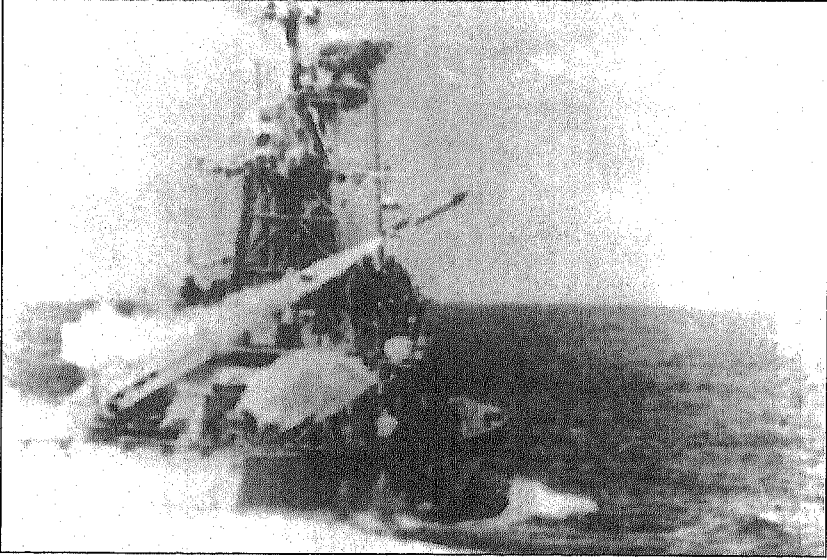
زورق صواريخ من طراز ريشيف Reshef يطلق صاروخه.
