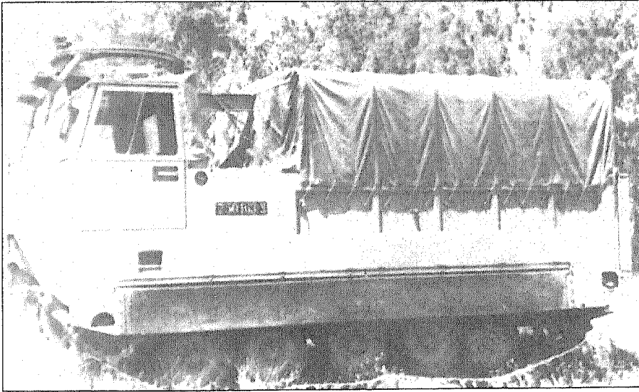
عربة نقل مجنزرة (طراز M548). تستخدم في نقل ذخيرة بطاريات المدفعية من عيار ١٥٥ مم و١٧٥ مم.
