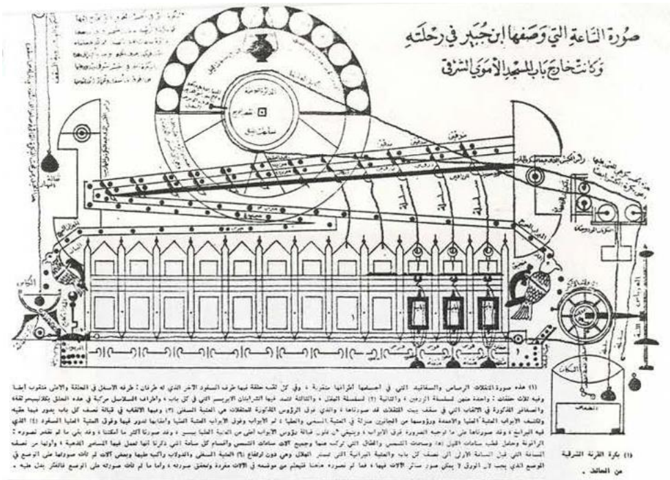
رسم الساعة التي وصفها ابن جبير كما رسمها ابن صانعها رضوان
