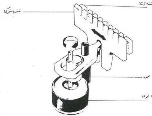
★ رأس المقص في الماكينة الهزازة الحركة ★
