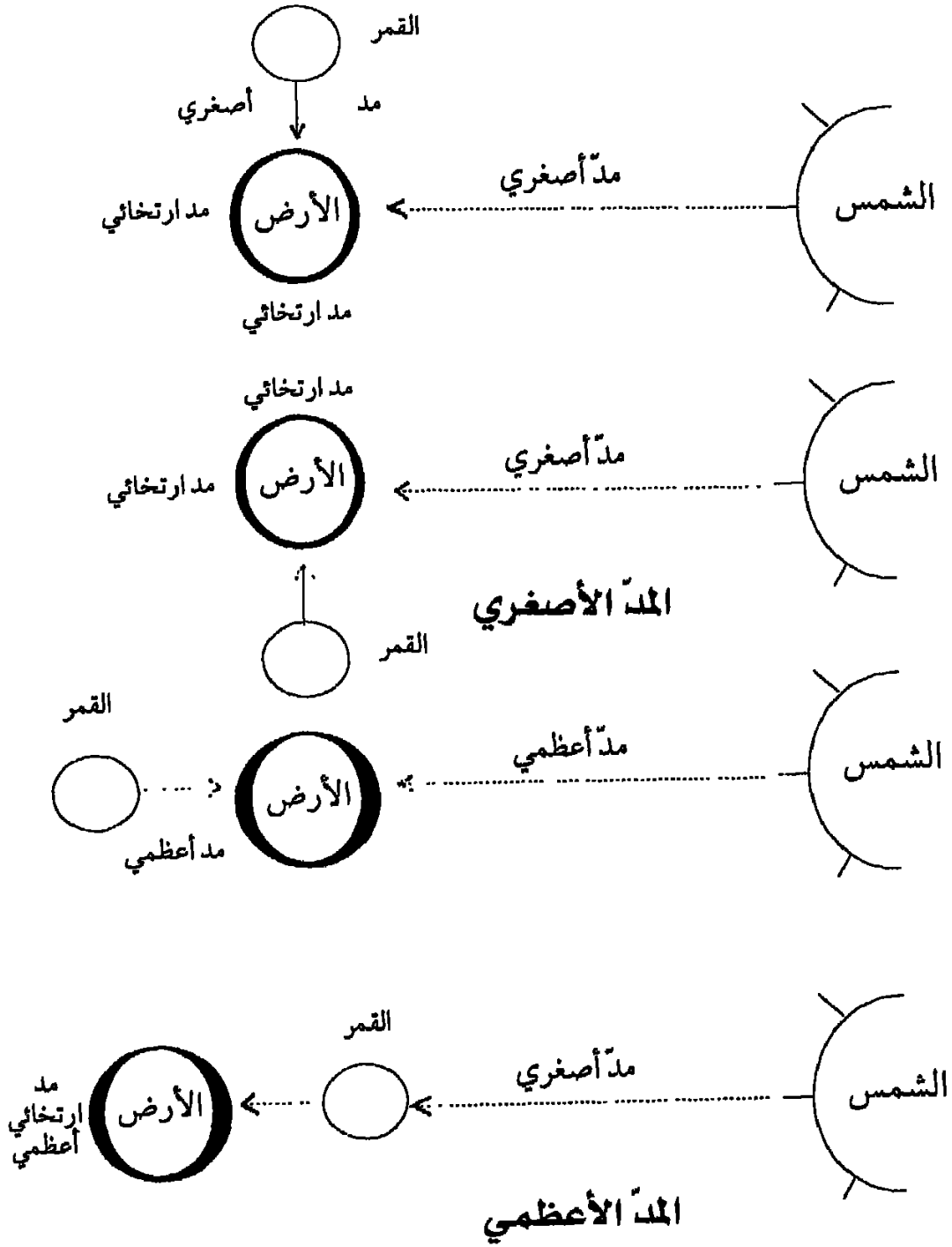
شكل ٦٤ أنواع المد والجزر في المحيطات والبحار والذي يعتمد حدوثه على مكان القمر حول الأرض
