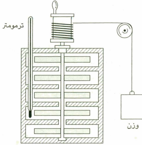
شكل ٤-٢: مخضة جول، الجهاز المستخدم لتحديد المكافئ الميكانيكي للحرارة.
