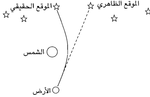
شكل ٦-١٥: الحيود الجاذبي لضوء نجم بواسطة الشمس.
