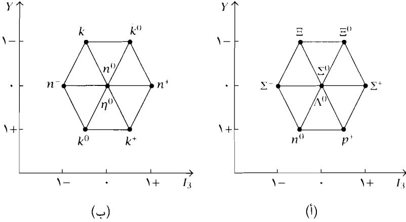
شكل ٨-٢: أشكال التقسيم. (أ) الدوران المغزلي ٢/١ للبريونات. (ب) الدوران المغزلي صفر للميزونات. Y الشحنة الزائدة. I_3 مكون Z - للدوران المغزلي النظائري.
