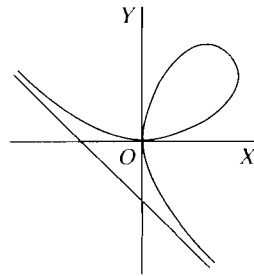
منحنى ديسكارتس
