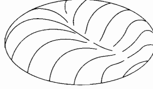
شكل ٧-١١: موجات ذات بعد واحد.
