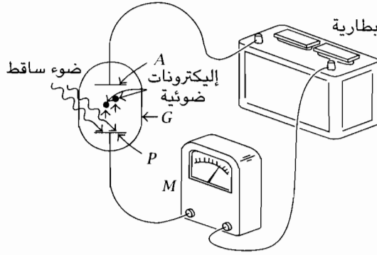
شكل ٥-٧: رسم تخطيطي للظاهرة الكهروضوئية. A أنود، P كاثود ضوئي، M جهاز لقياس التيار، G مصباح زجاجي مفرغ من الداخل.
