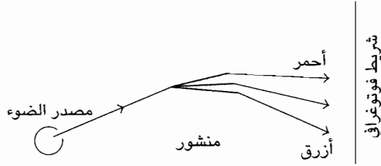
شكل ٧-٨: تشتت الضوء إلى طيف. يتشتت الضوء من المصدر بواسطة المنشور إلى طيف من الألوان (ترددات)، يتم تسجيلها على شريط فوتوغرافي.
