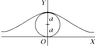
منحنى أجنيسي
