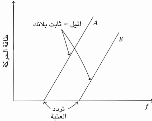
شكل ٧-٦: تنبؤ أينشتاين بالعلاقة بين طاقة الفوتوإلكترون القصوى والتردد. KE طاقة الحركة القصوى للفوتوإلكترون، f تردد الضوء الساقط، A, B مادتان مختلفتان، Thr حد التردد.
