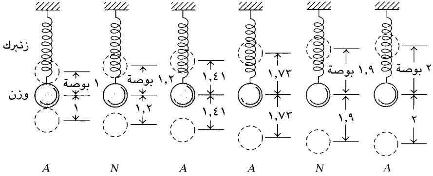
شكل ٧-٤: ساعات المتذبذب. A مسموح، N غير مسموح.
