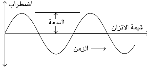
شكل ٧-١٣: خصائص الموجات.
