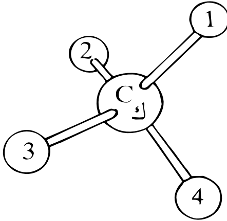
التوزيع الفراغي للروابط الأربعة حول ذرة الكربون
