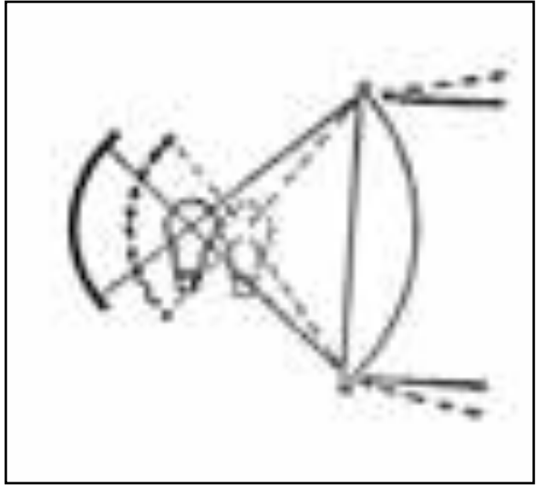
(٩٨) قرب اللمبة بالمرآة المقعرة العاكسة خلفها - من العدسة الفريزنييل ويبعدها عن العدسة، هي أهم شيء في إرسال الضوء إلى مسافة أبعد
